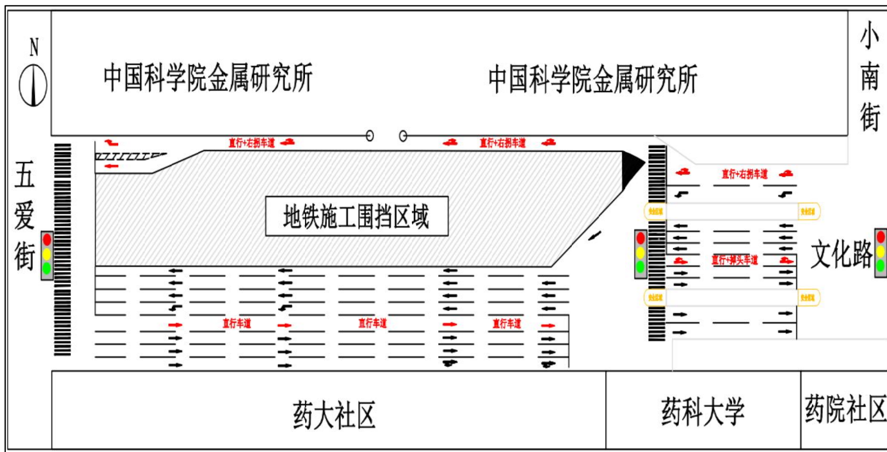
导流图一
