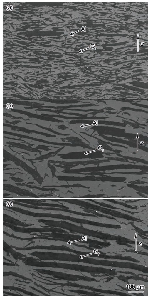
图3 不同尺寸片层石墨G r /Al复合材料的SEM像 Fig.3 SEM images of graphite flake G r /Al composites in different sizes (a) 150 μm (b) 300 μm (c) 500 μm
