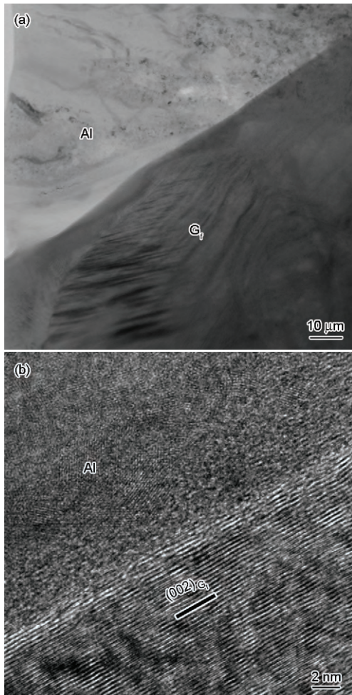
图5 500 \mu m 片层石墨 G_r/Al 复合材料界面的TEM和HRTEM像
