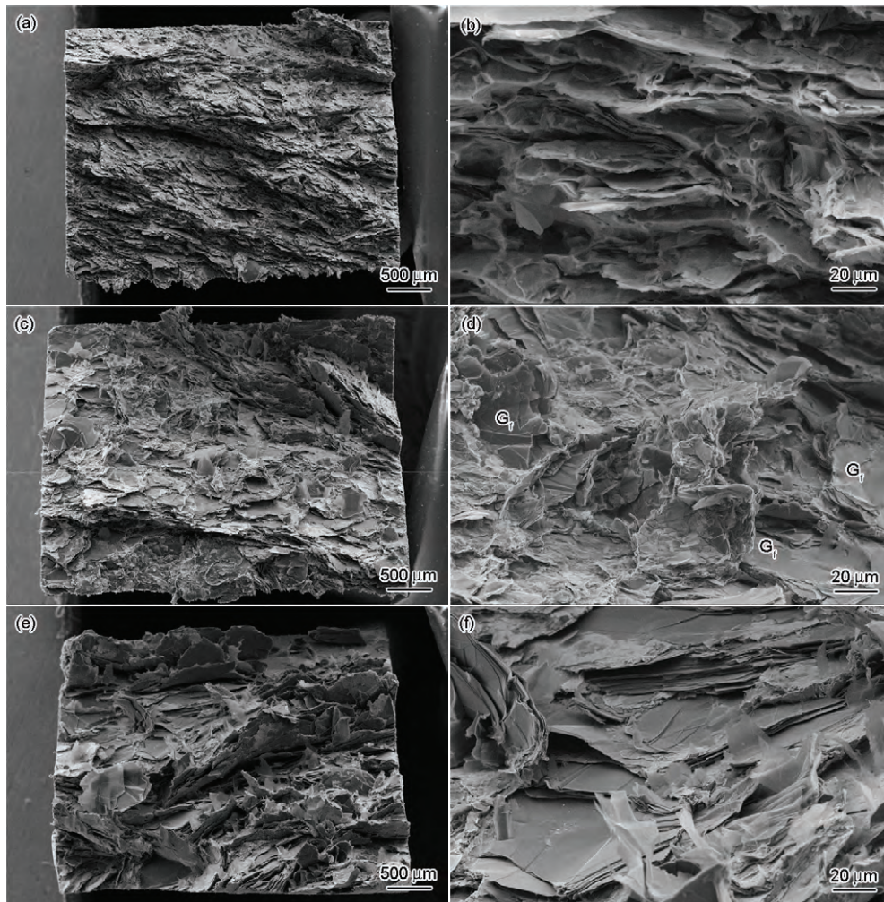
图6 不同尺寸片层石墨 G_r /Al 复合材料断口的 SEM 像
