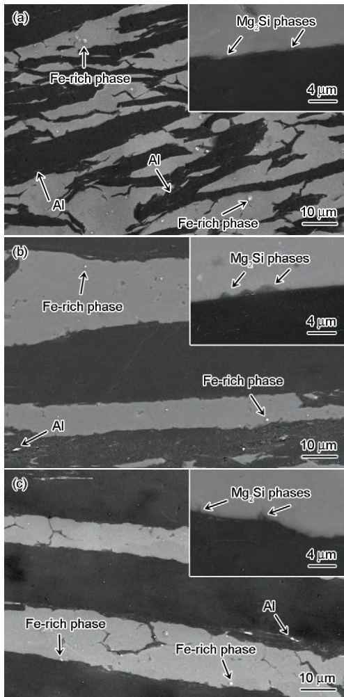
图4 不同尺寸片层石墨 \text{G}_r/\text{Al} 复合材料的放大SEM像
